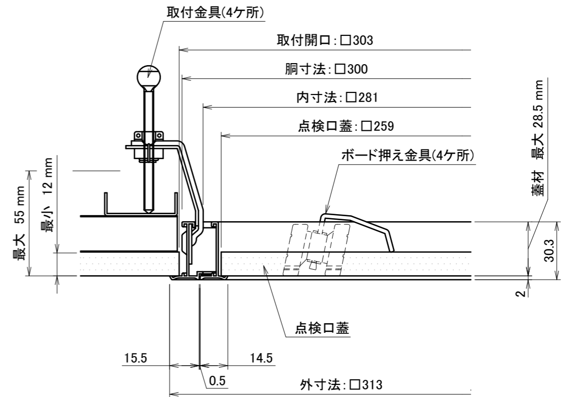
軽鉄下地の場合 (S=1/2)
