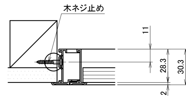
木下地の場合 (S=1/2)
