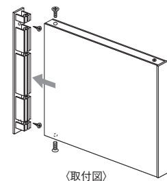
(取付図)
